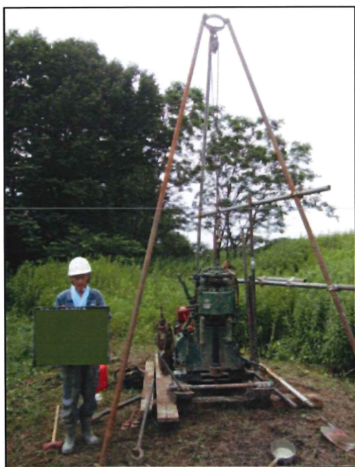
ボーリング調査の例
