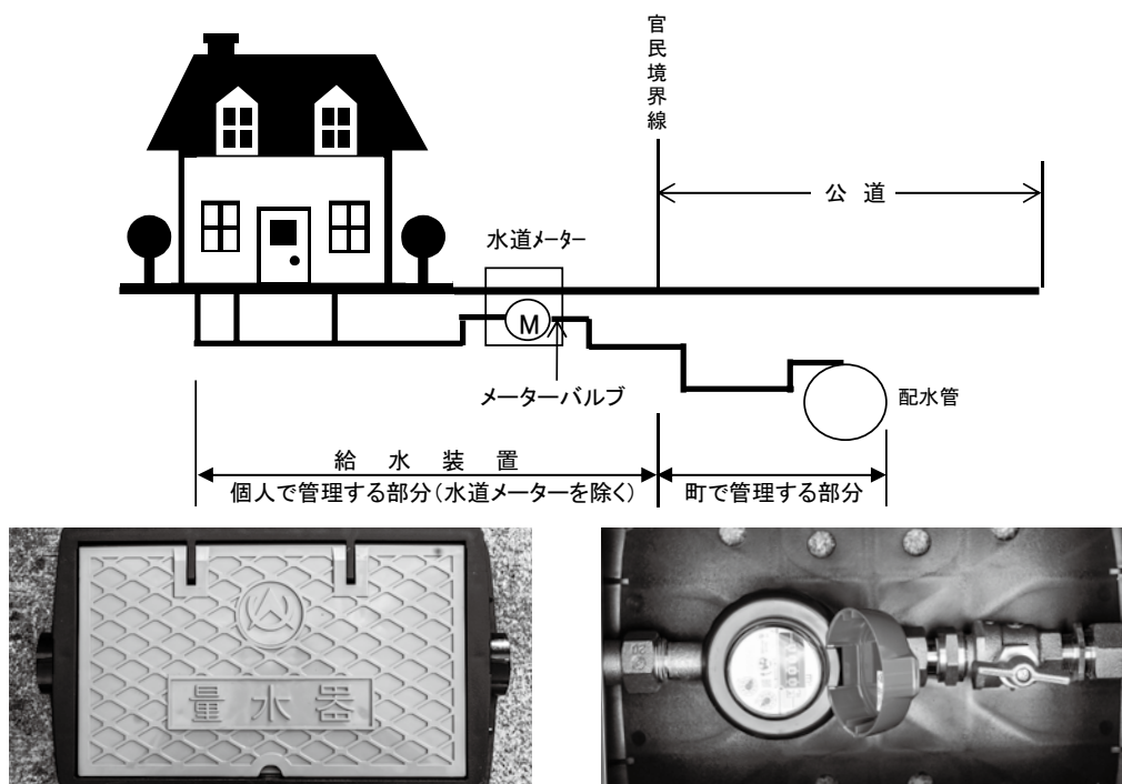
一般的な水道メーターボックス
