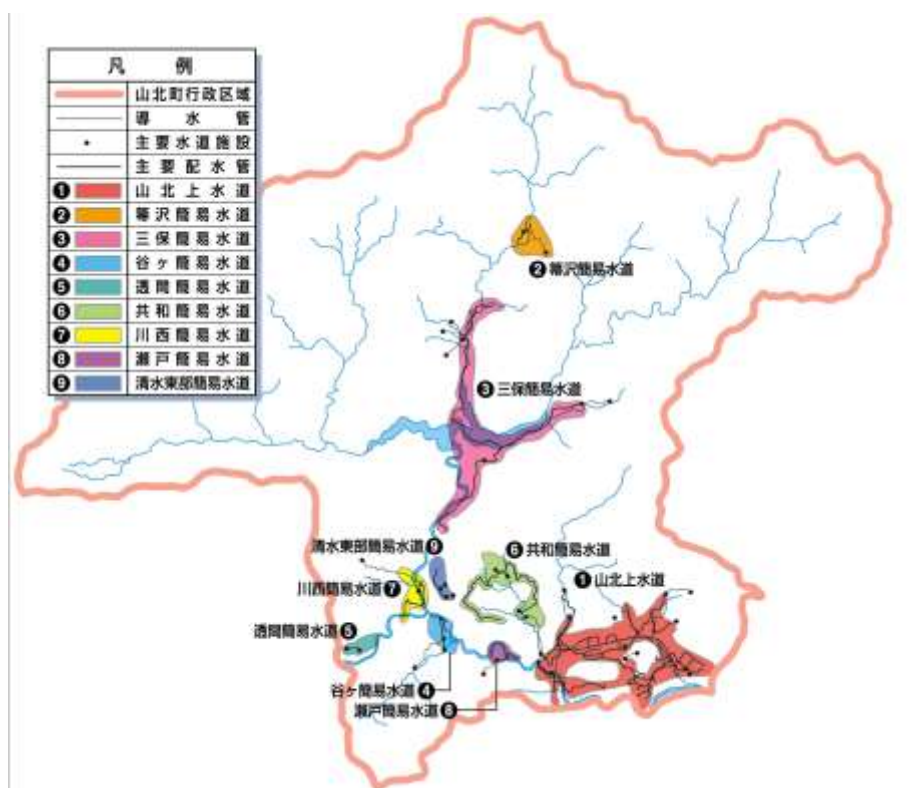
図2 上水道及び簡易水道概略図
