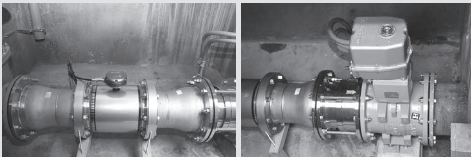
更新された緊急遮断弁（写真右）と流量計
