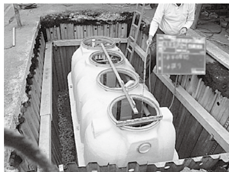
高度処理型合併処理浄化槽設置の様子
